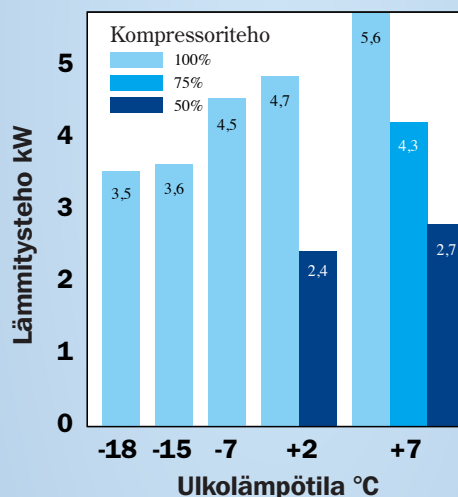
Lämmitysteho
