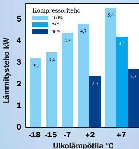
Lämmitysteho
